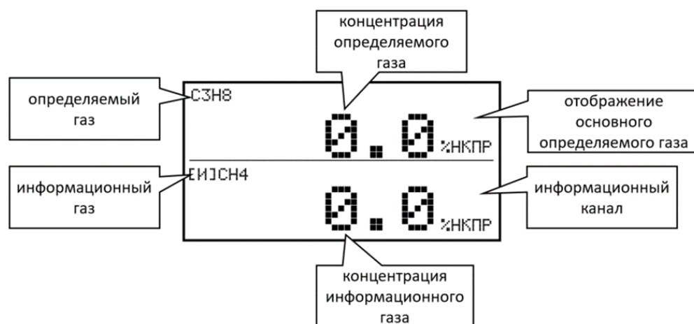
Рисунок 36 – Отображение информационного канала
