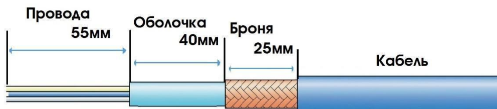
Рисунок 21 – Подготовка кабеля с бронезащитой
