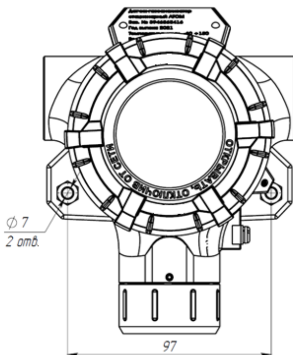
Рисунок 25 – Монтажные размеры
