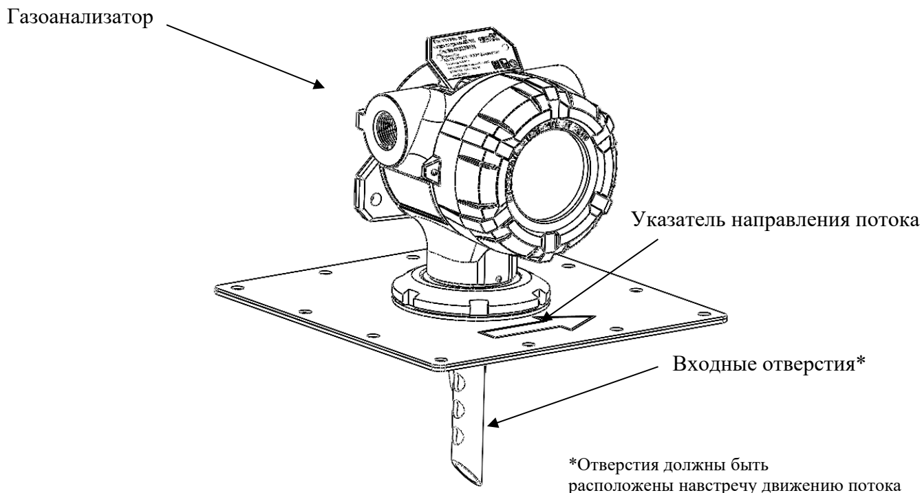
Рисунок 31 - Внешний вид газоанализатора и комплекта для монтажа в воздуховоде
