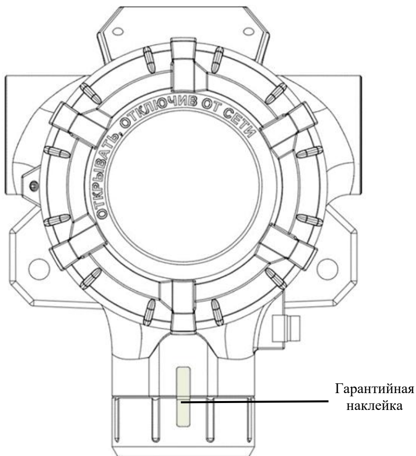
Рисунок 15 – Пломбировка узлов газоанализатора
