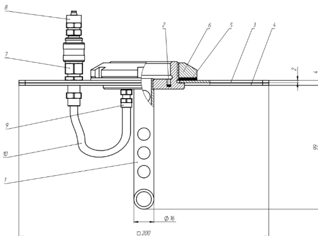
Рисунок 30 - Общий вид комплекта.
