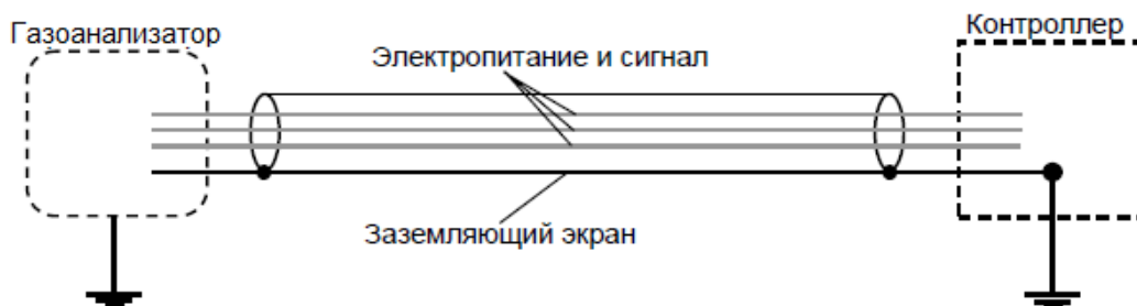
Рисунок 24 – Заземление экранированного кабеля
