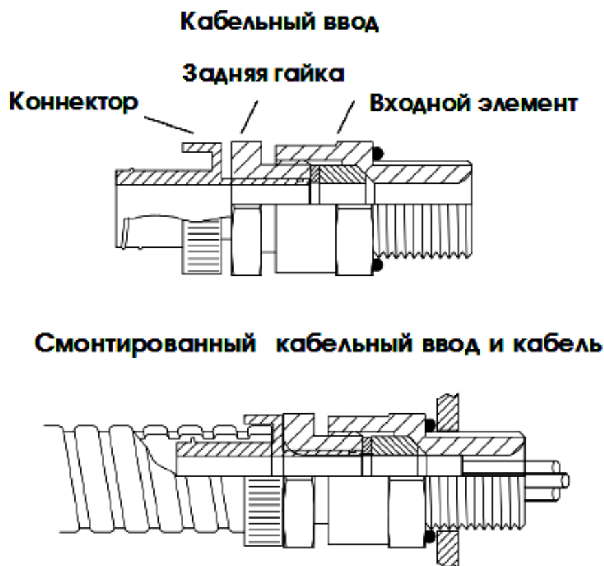
Рисунок 18 – Монтаж кабельного ввода
