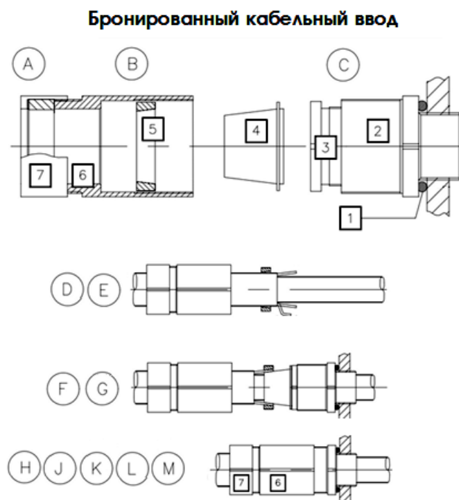
Рисунок 20 – Монтаж кабельного ввода с бронезащитой
