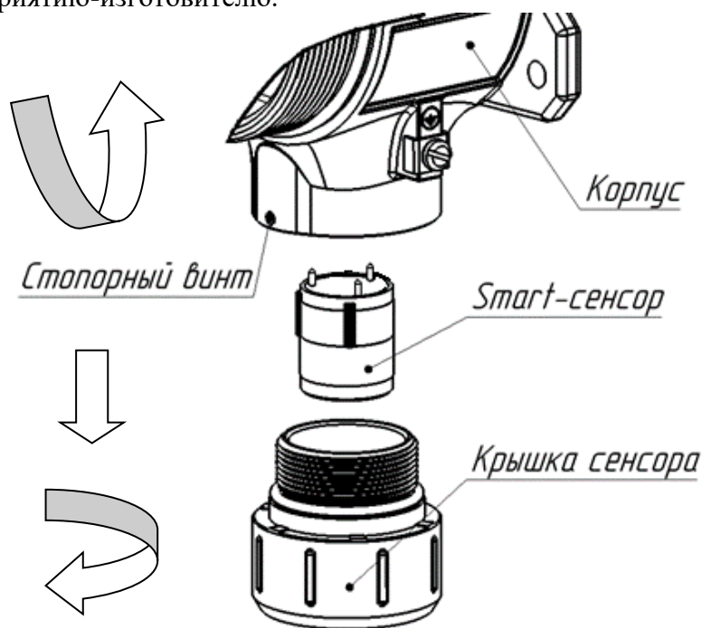
Рисунок 43– Схема разборки при замене сенсора
